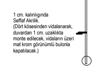
YAN GÖRÜNÜŞ DETAYI Ö :1/10
